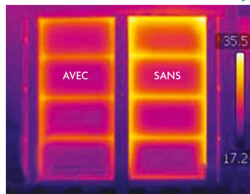
Chambre de test avec 2 échantillons de portes assemblées : - à gauche : panneau Thermalsafe double-coque de 40 mm - à droite : panneau série mono-coque de 40 mm Plus la couleur est jaune, plus la déperdition de chaleur se fait sentir.
