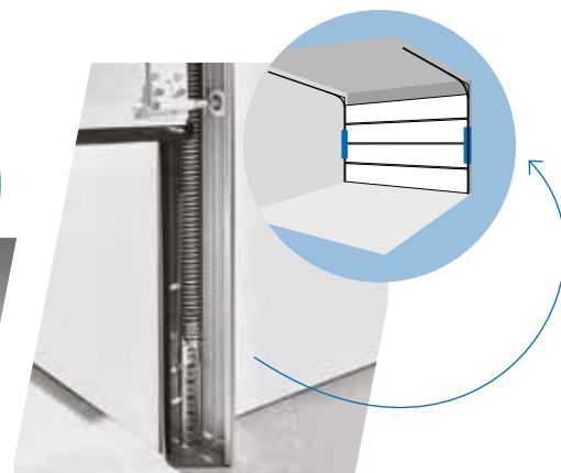
ATTRACTIVE : ressorts à traction
